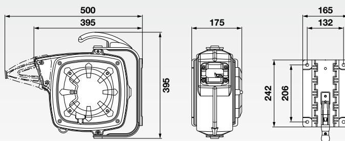
Габаритные размеры катушек с кронштейном (мм)
