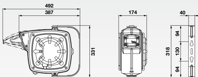
Габаритные размеры стандартных катушек (мм)
